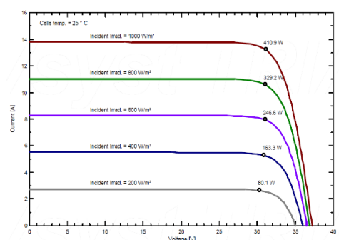
Curva I-V dei moduli (SPV41x-R54JWML)
